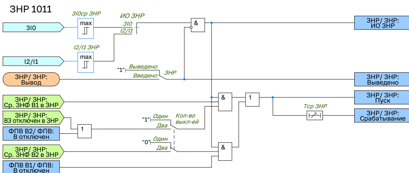
Рисунок 1.34 – Функциональная схема ЗНР
