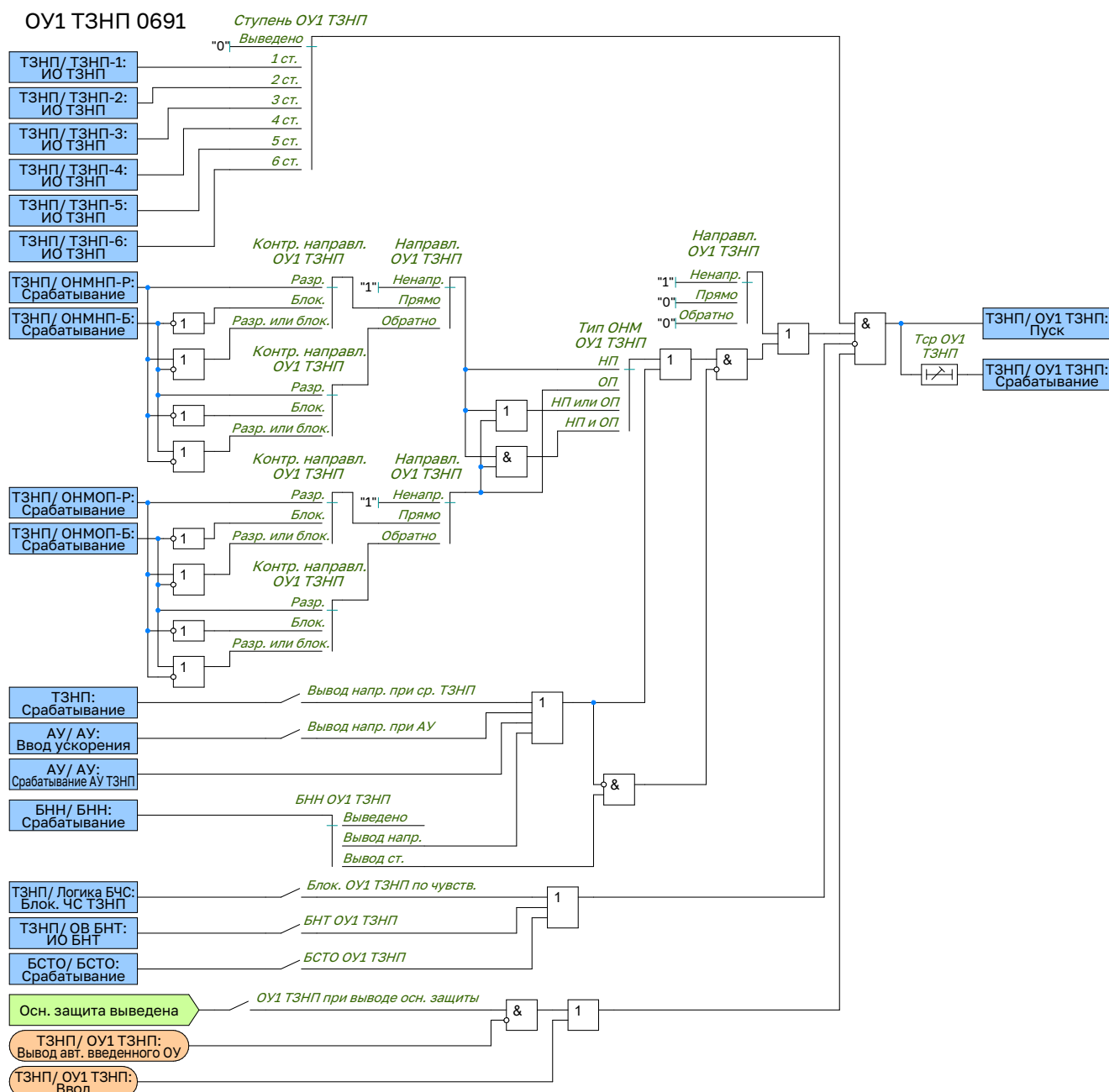
Рисунок 1.26 – Функциональная схема ОУ ТЗНП
